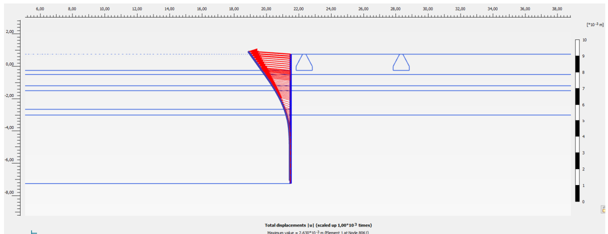
verplaatsing damwand stage 4 - ontgraving stempelraam
